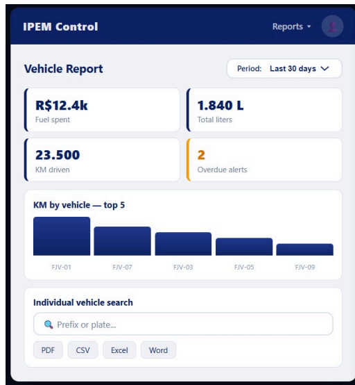
Imagem 16 – Relatório de Viaturas
